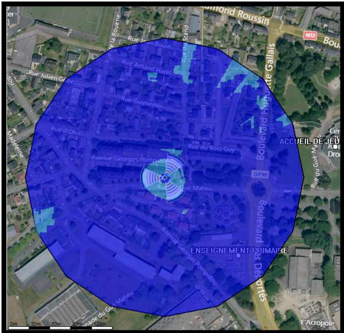
Fond de carte (photo aérienne), source : bing. Logiciel de simulation Cellergy, éditeur Orange Labs
